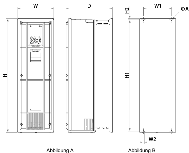
Externe Abmessungen des Umrichters (Standard)
